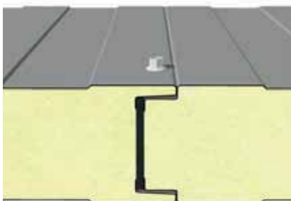
Detalle del sistema de fijación
